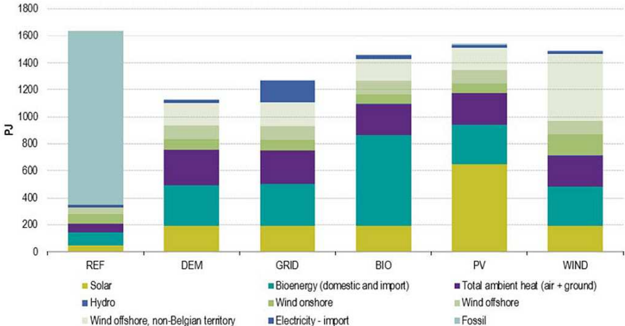
Figuur EX1: Primaire energievraag, alle scenario's, 2050 (PJ)
